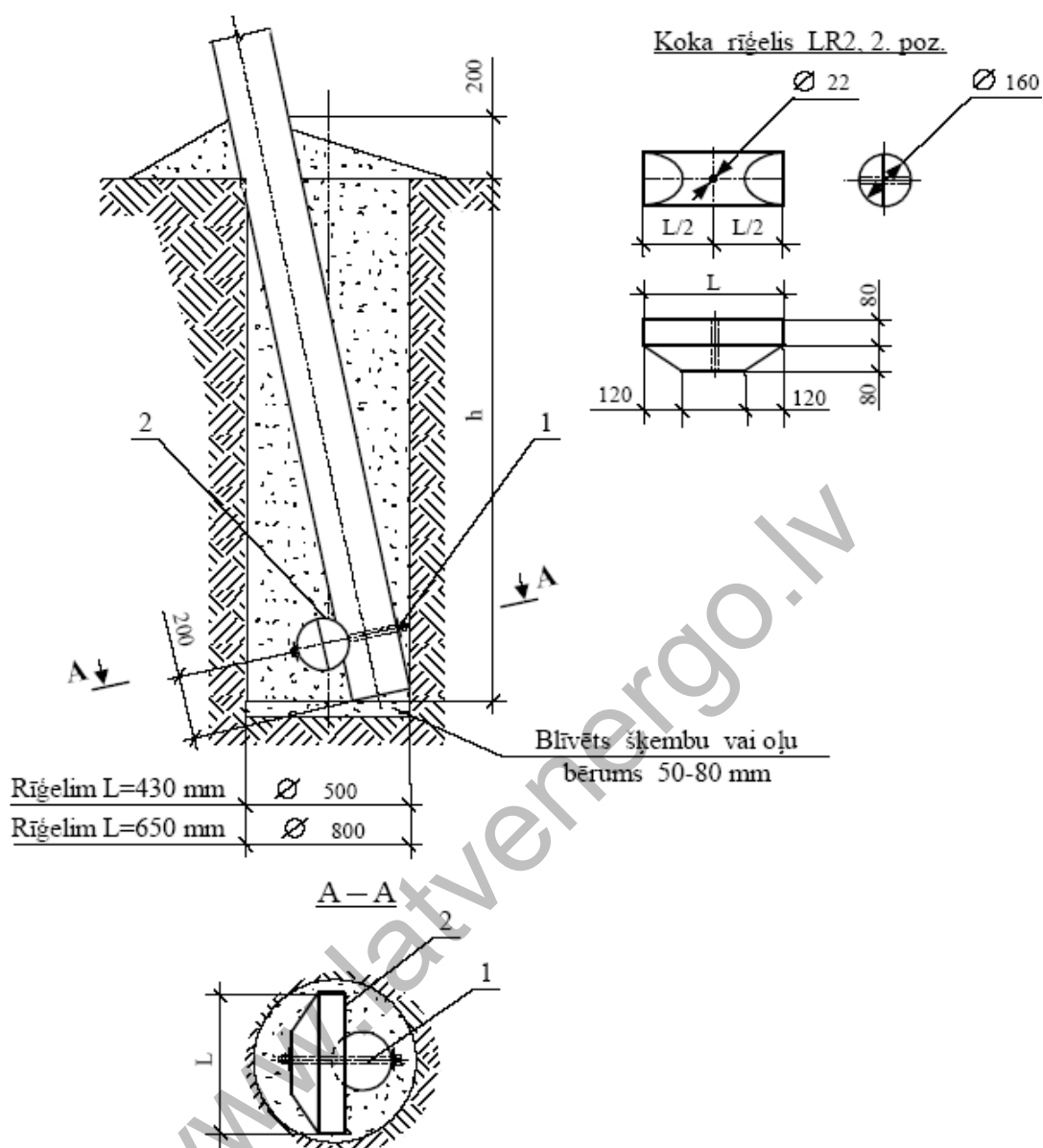
5.2. attēls. Statņa nostiprināšana gruntī ar vienu apakšējo rīgeli
