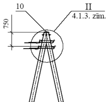
Stūra starpbalsts SSA04P.4s (pārējo sk. stūra starpbalstu SSA04P.4n)
