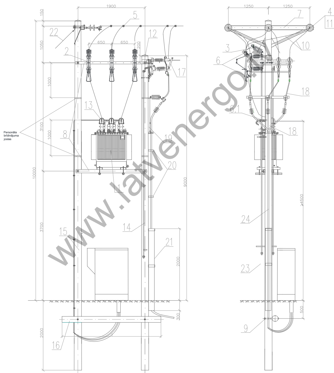
5.7. attēls. Apakšstacijas ar drošinātājtaldlītāju un vienu komutējamu 20 kV kabelpievadu TA 20/0,4.630P-GDAG +1K konstrukcija
