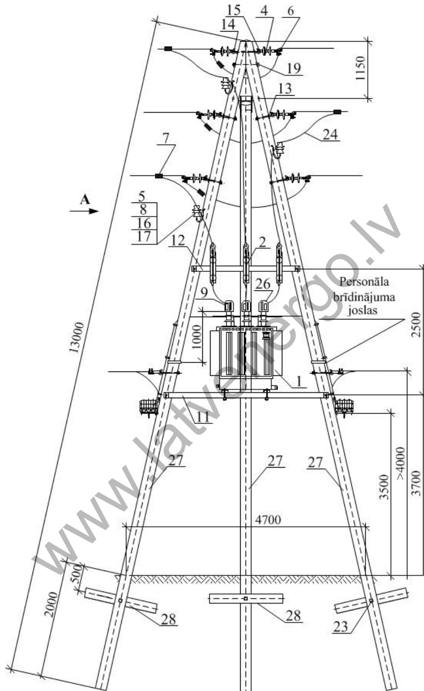
7.3. attēls. Caurejošās 3 kāju balsta apakšstacijas TA 20/0,4.250T-SDA konstrukcija
