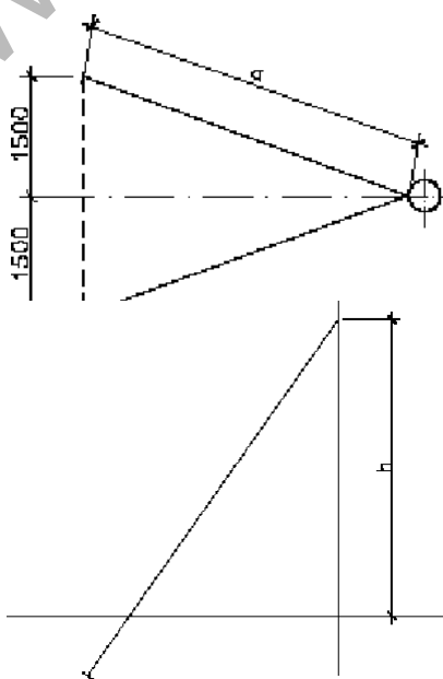
8.3. attēls. Atsaišu uzstādīšana un atsaišu izmēri vienstatņu balstam
