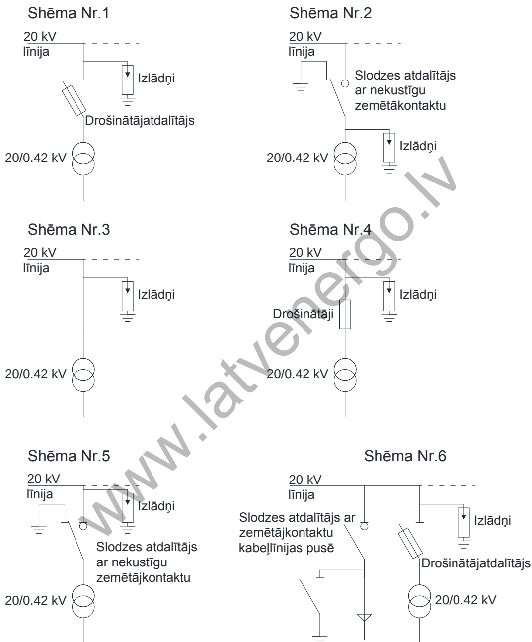
2.1. attēls. Mastā apakšstaciju 20 kV puses shēmas
