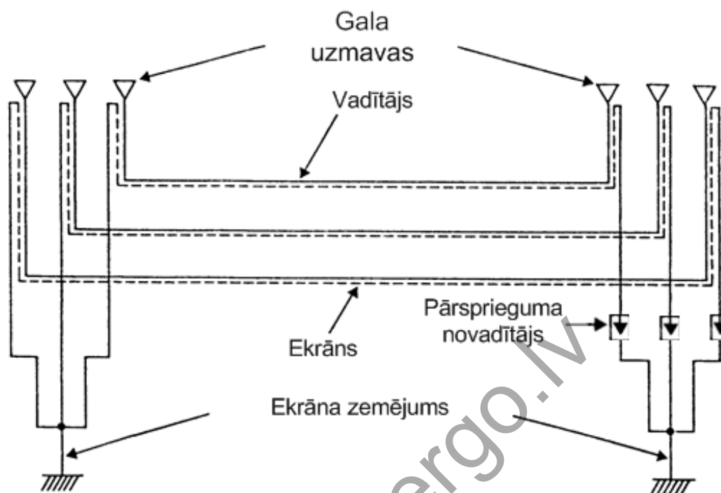
5.2. attēls. Ekrāni zemēti viena kabeļa galā
