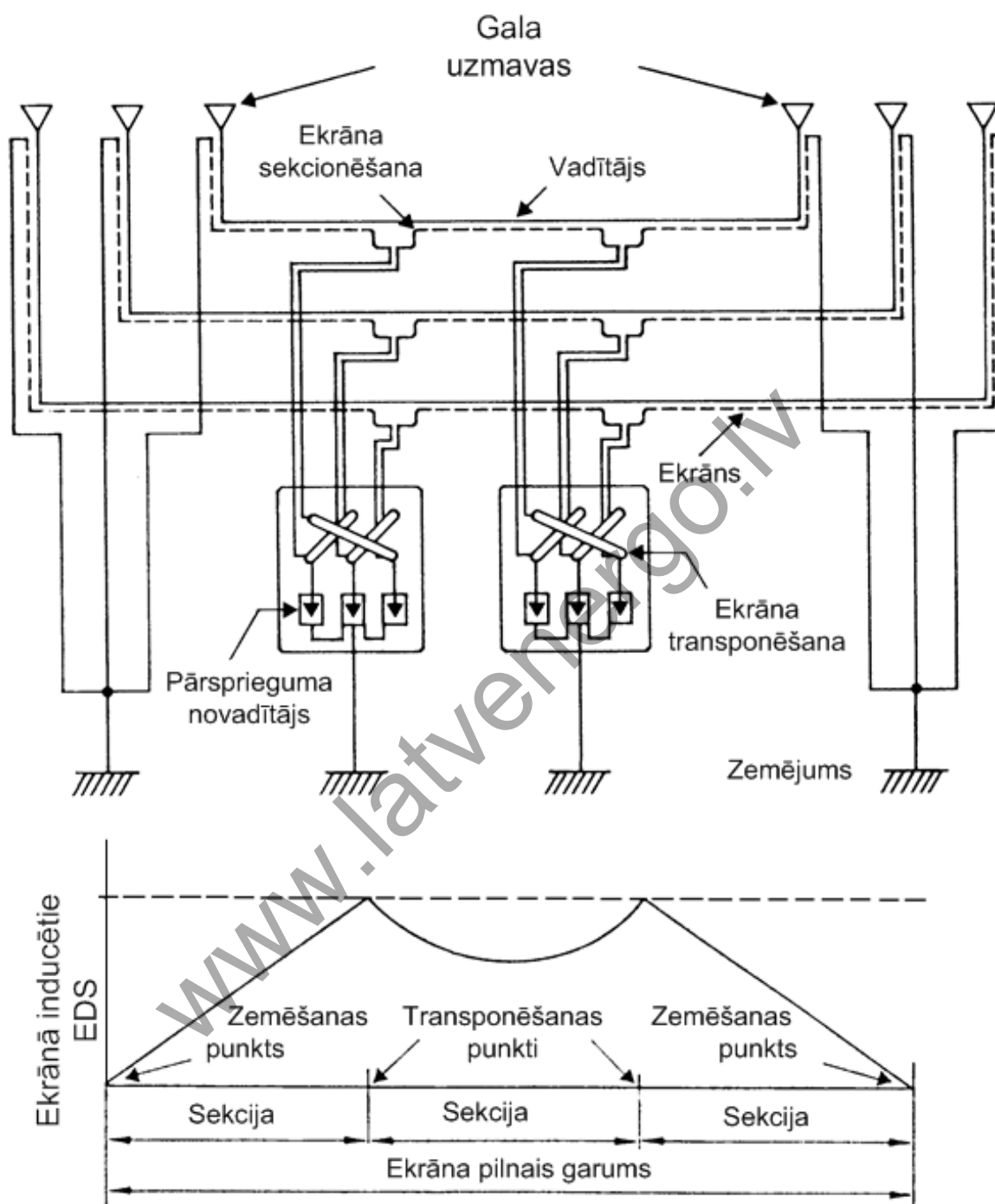
5.4. attēls. Ekrānu transpozīcija. Inducēto EDS diagramma
