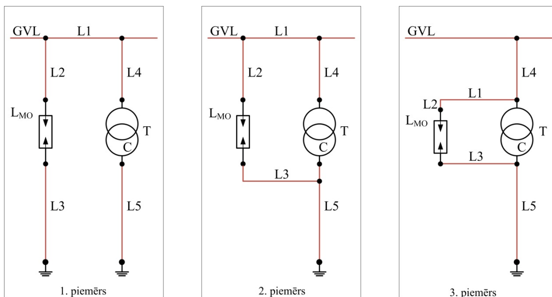
2.1. attēls. PAI pievienojuma piemēri
