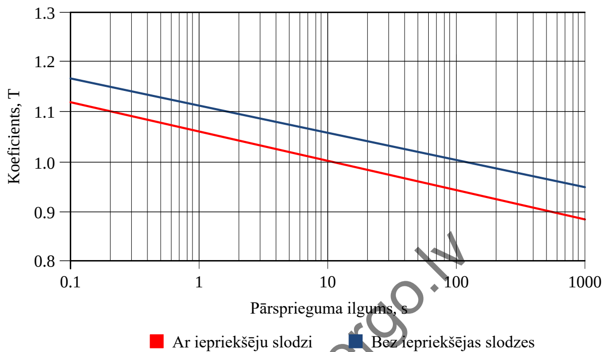
P3. 1. attēls. TOV raksturlīkne atkarībā no PAI nominālā sprieguma ( U_r )
