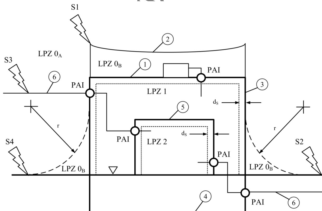
4.2. attēls. Zibensaizsardzības zonu koncepcija aizsargājamam objektam
