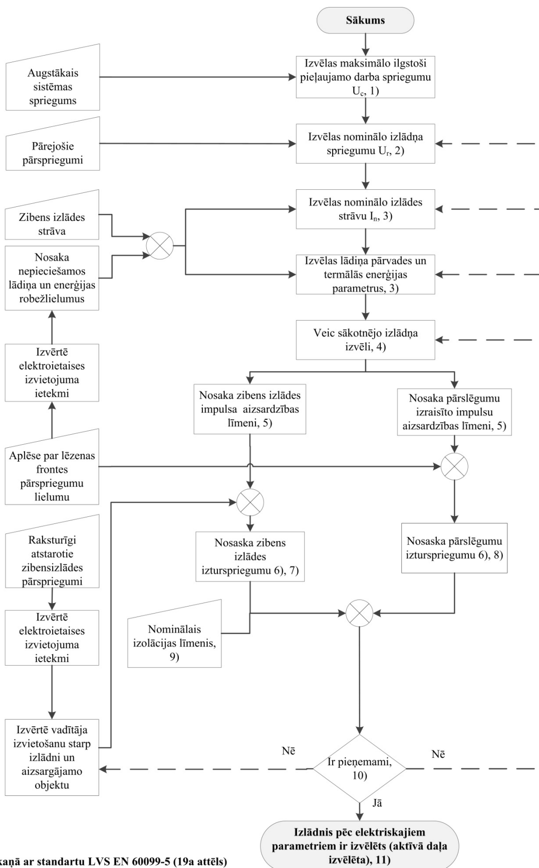
P1. 2. attēls. PAI izvēle pēc elektriskajiem parametriem.
