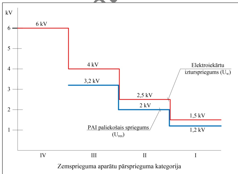
4.1. attēls. Aizsardzības līmenis (paliekošais spriegums) 230/400 V elektrotīklā
