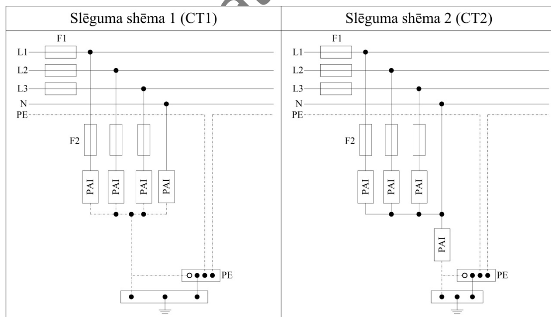
4.3. attēls. PAI slēguma shēmas
