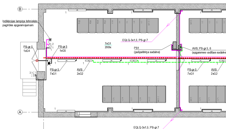
7.7. attēls. Apakšstaciju un sadales punktu apgaismes tīkla marķējums
