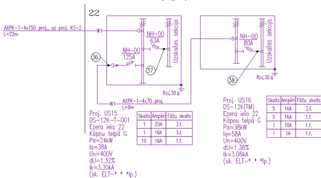
Attēls 5.12. Uzskaites sadalņu kabeļu sekciju attēlojuma piemērs.
