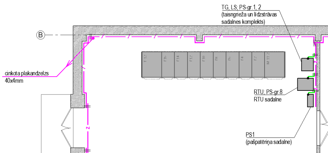
7.8. attēls. Apakšstaciju un sadales punktu zemējum tīkla marķējums
