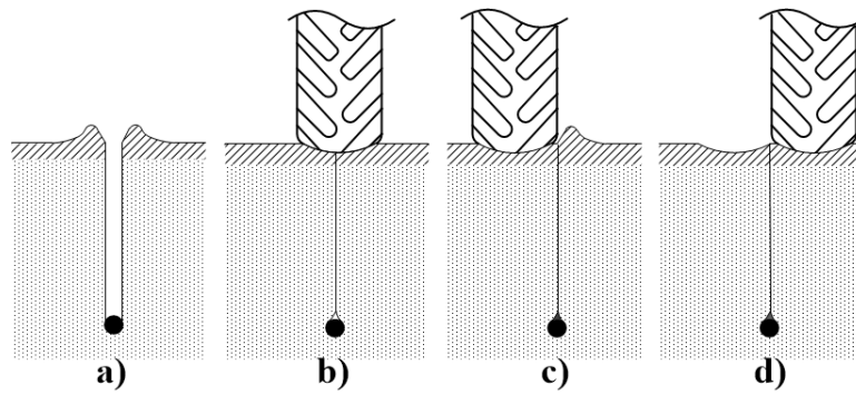
P1.13. attēls. Piemērs tranšijas blīvēšanas secībai
