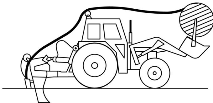
P1.5. attēls. Kabeļa saivas novietojums uz riteņtraktora
