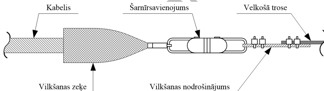
P1.6. attēls. Vilkšanas nodrošinājums
