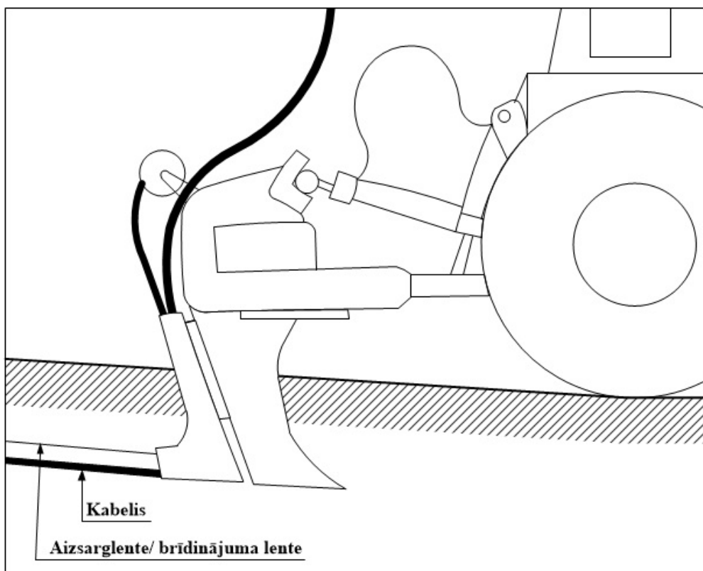
P1.7. attēls. Aizsarglentes un brīdinājuma lentes ieguldīšana ar kabelārklu
