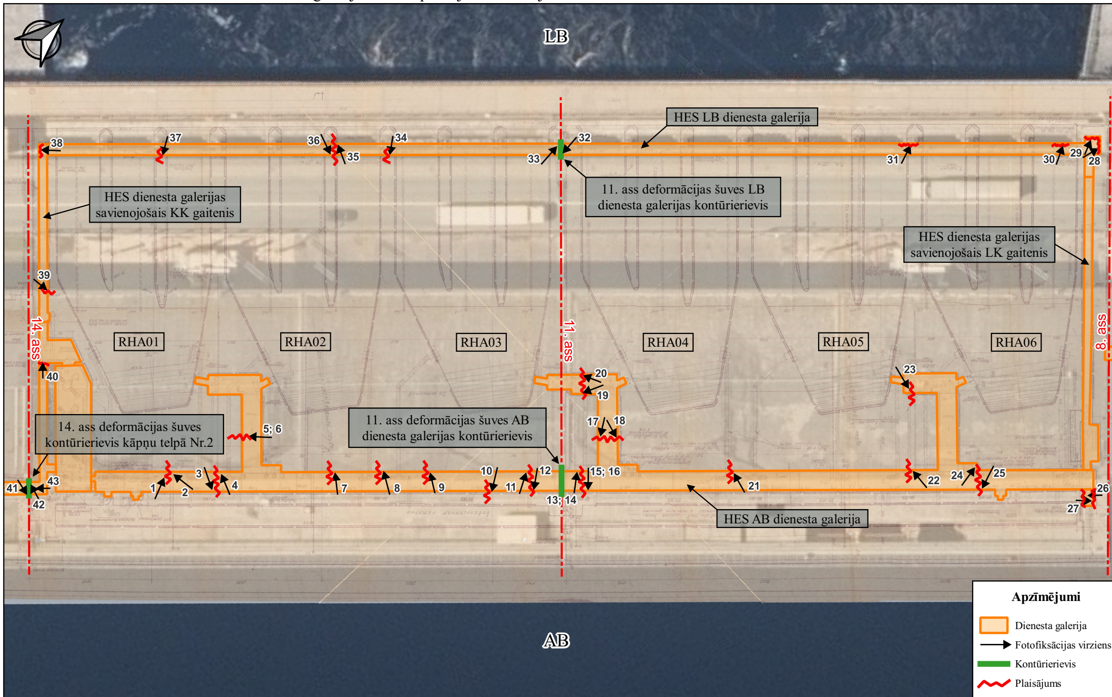
▼ Shēma Nr.1 - HES ēkas AB un LB dienesta galerijās fiksēto plaisājumu izvietojuma shēma
