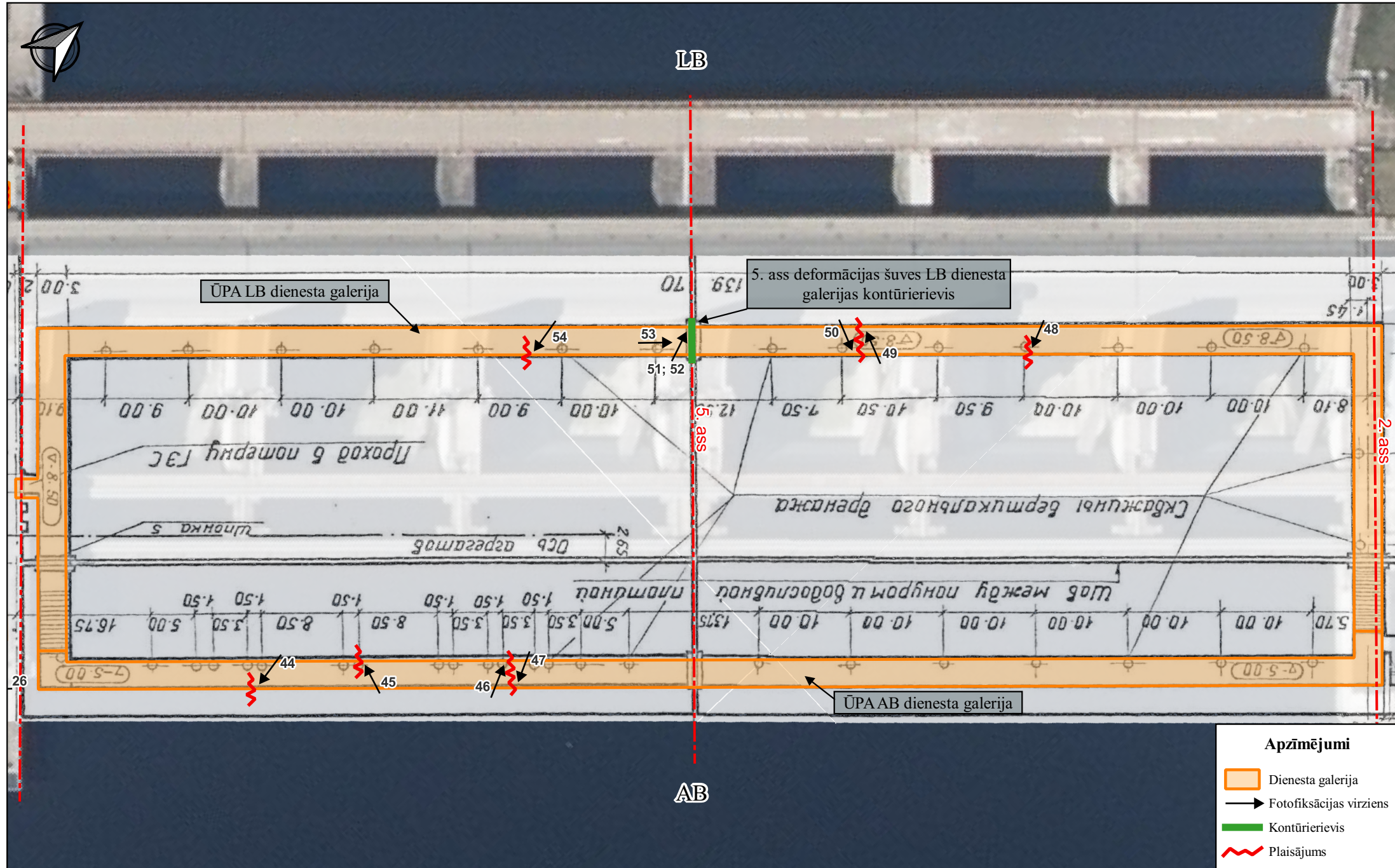
▼ Shēma Nr.2 - ŪPA AB un LB dienesta galerijās fiksēto plaisājumu izvietojuma shēma
